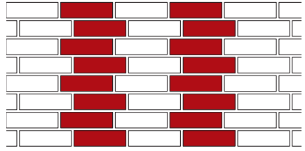
Ложковая в четверть кирпича
