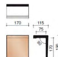
Пультовая моночерепица 90°
