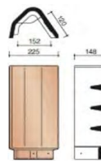
Пультовая черепица
