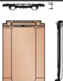
Двухволновая черепица
