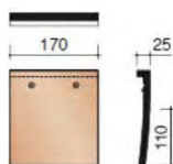
Карнизная/верхняя
