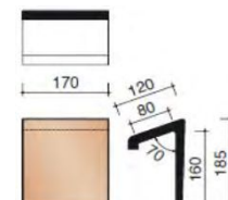
Пультовая моночерепица 70°
