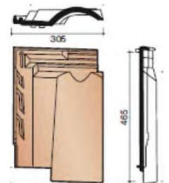
Подконьковая черепица
