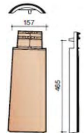
Черепица 1/2
