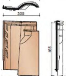
Вентиляционная черепица
