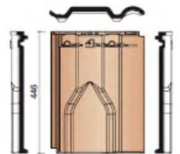
Вентиляционная черепица
